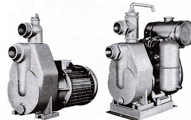
Selbstsaugende Baupumpe mit Elektromotor
