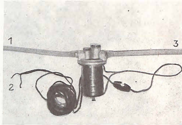
1 Anschlußstück zum eigenen Behälter, 2 Anschlußstück zu den beiden Batterien, 3 Anschlußstück zum fremden Behälter
