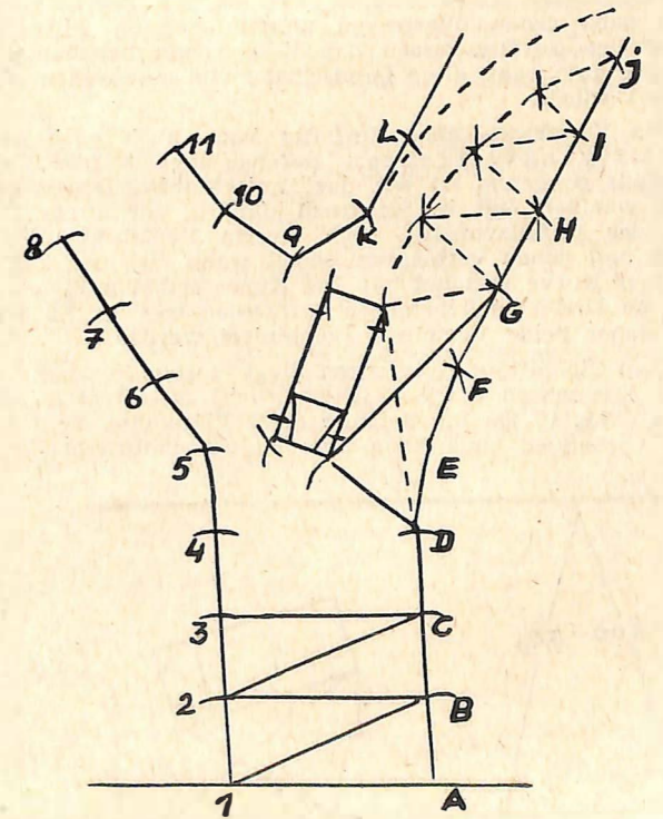
Abb. 2 Dreiecksmessverfahren, kombiniert mit Schnittpunktverfahren bei Kurven und Einmündungen
