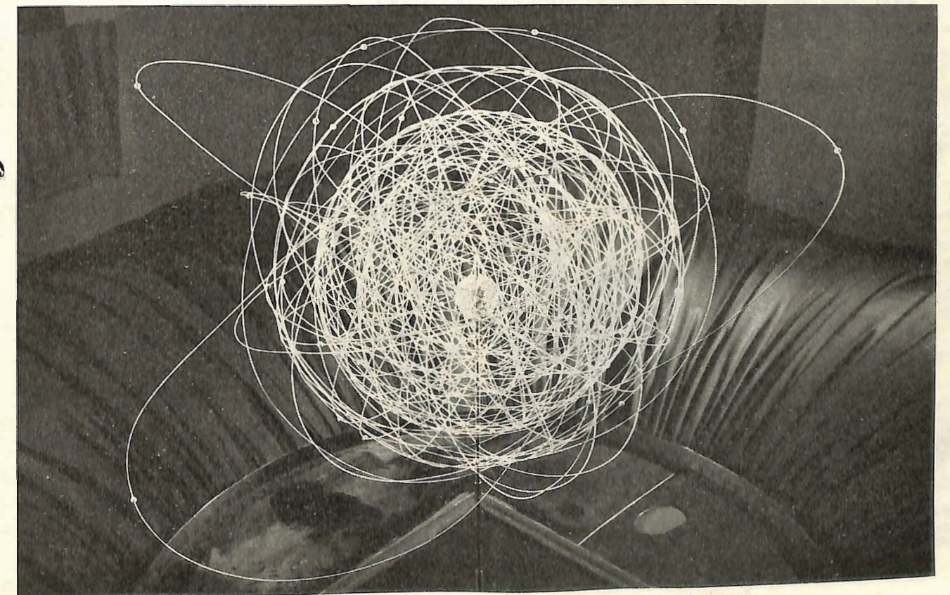
Modell eines Uranium-Atoms. In der Mitte der Kern, um ihn herum die Bahnen der 92 Elektronen
