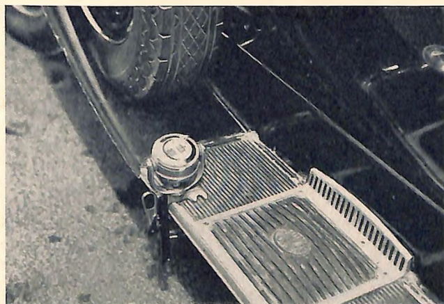
Ebenfalls ein Bremsmesser, jedoch englisches System Tapley. Diese Apparate ermöglichen eine genaue Kontrolle des Zustandes der Bremsvorrichtungen.
