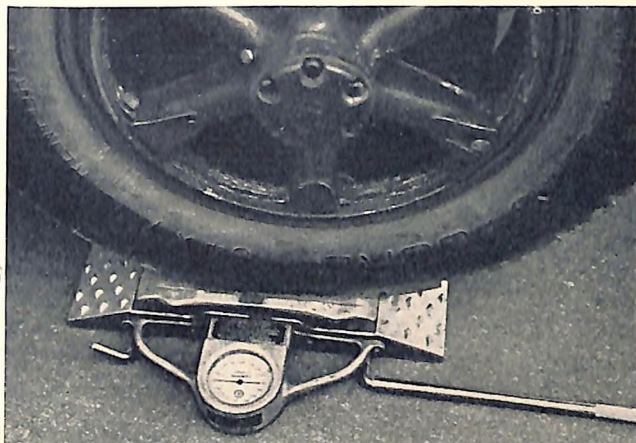
Ein Gerät zur Überprüfung des Wagengewichtes. Das Auto fährt erst mit dem vorderen Räderpaar auf zwei Gewichtsmesser und hernach mit dem rückwärtigen Räderpaar. Die Gewichtsangabe erfolgt bis auf 20 Kilogramm genau.
