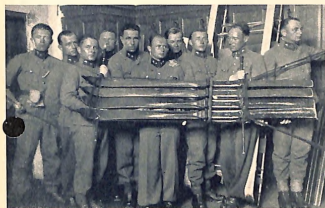
Die Frequentanten der Gendarmerie-Akademie mit einem von ihnen gebauten Bilgeri-Rettungsschlitten. Ein solcher Schlitten kann nur mit Skiern mit Bilgeri-Bindung geschaffen werden, da sich andere Bindungen infolge ihrer Bauart hierzu nicht verwenden lassen.
