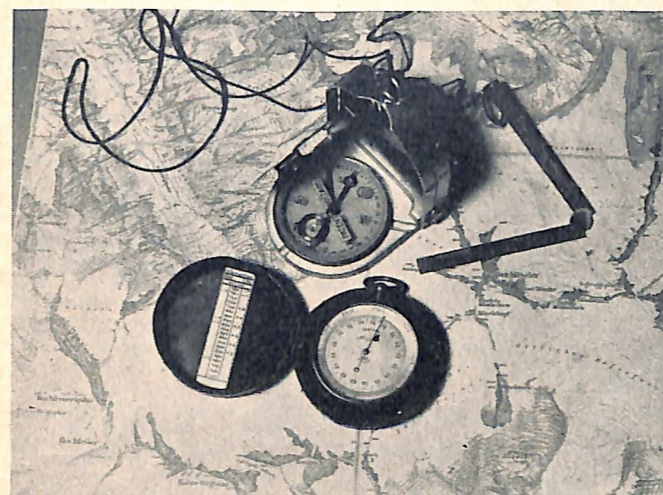
Die Orientierungsmittel des Gendarmen im Hochgebirge: Karte (hier die neue Alpenvereinskarte 1 : 25.000), Bézardbuffole mit Lineal, Pendel und Libelle, kompenzierter Höhenmesser.
