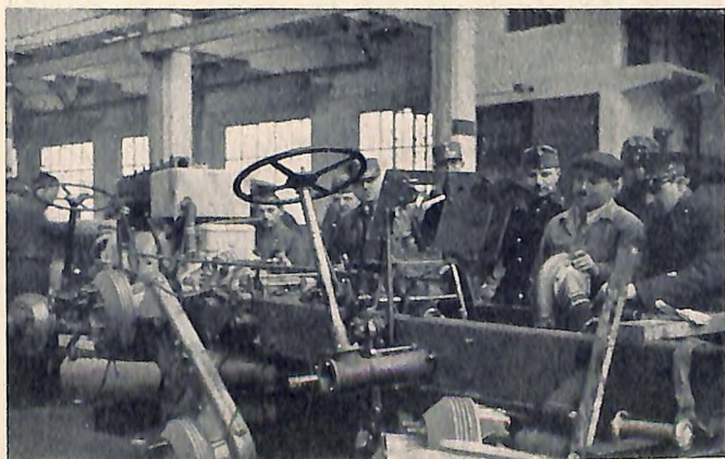
In der Montagehalle. — Wie der Panzerwagen entsteht.
