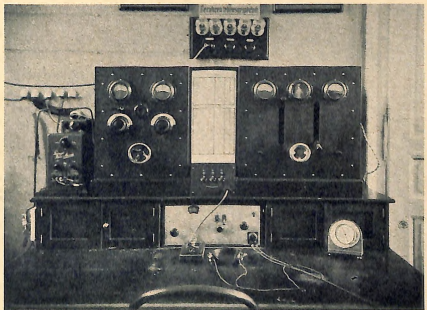
75 Watt-Sender samt Empfänger bei der Gendarmeriehauptfunkstelle.
