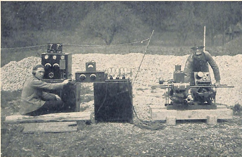
Mobile Funkanlage in Tätigkeit auf freiem Felde.
