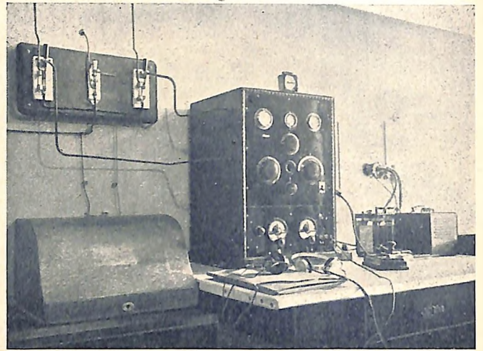
10 Watt-Sender samt Empfänger, Normaltype der Gendarmeriefunkstellen.
