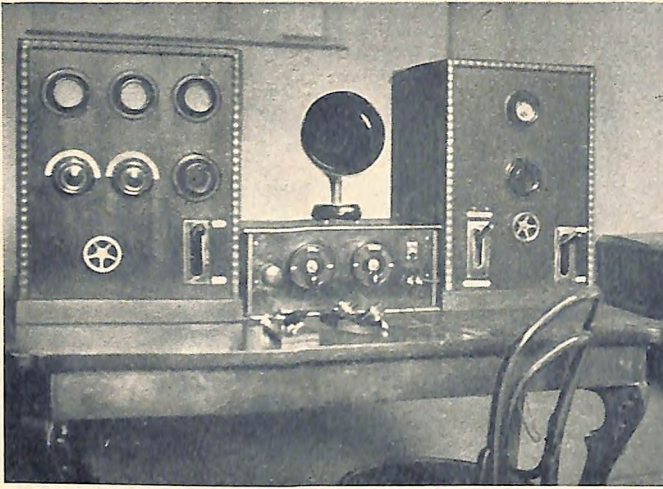
40 Watt-Sender samt Empfänger, Normaltype, bei den Gendarmerieleitfunkstellen.
