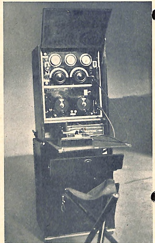
Von zwei Mann tragbare Sende- und Empfangsanlage.
